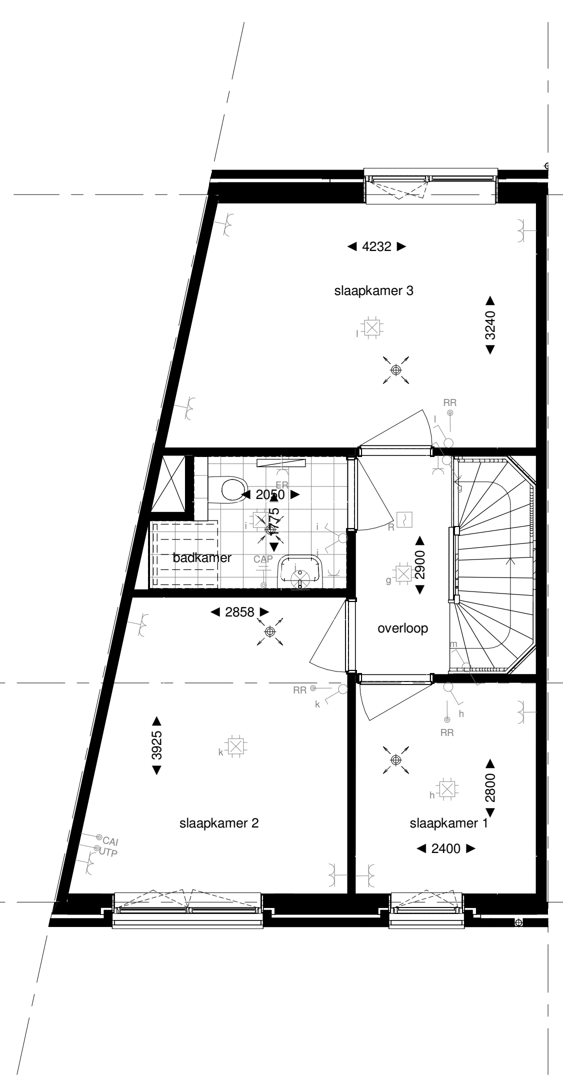
1e verdieping 1 : 50
