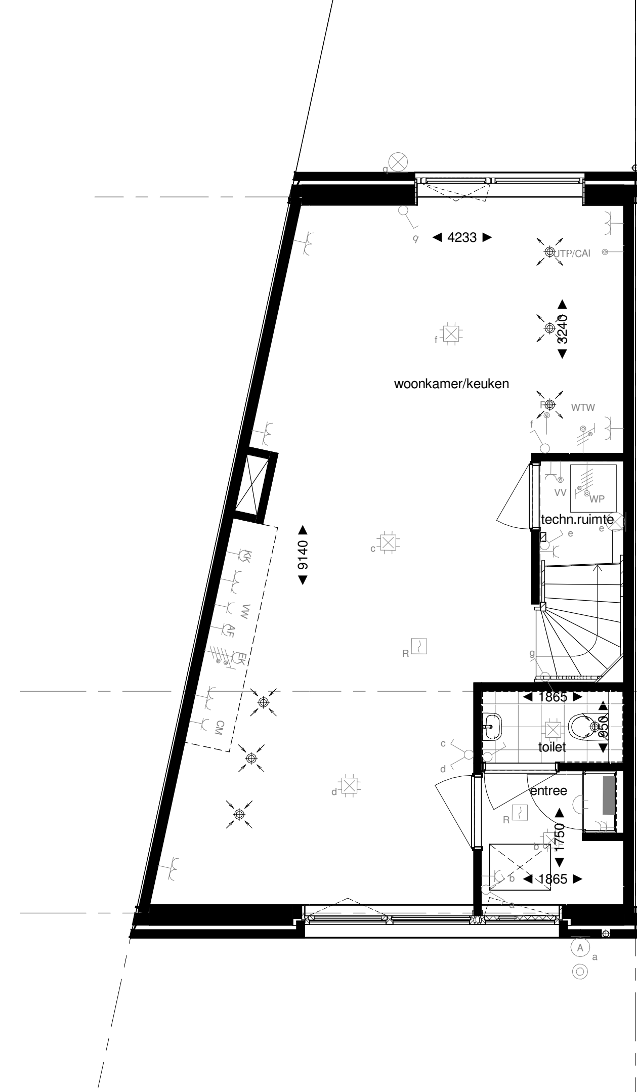
begane grond 1 : 50
