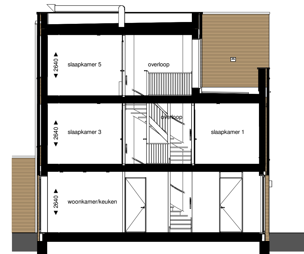
doorsnede 1 : 100
