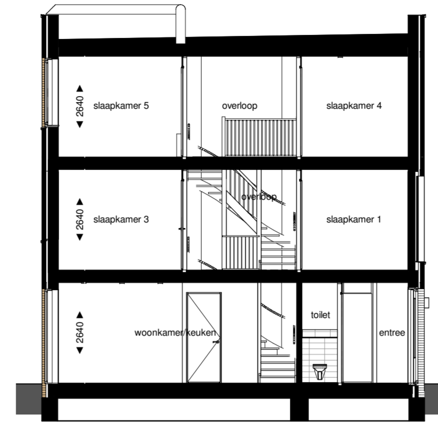
doorsnede 1 : 100
