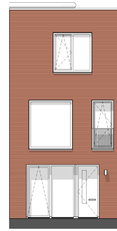
voorgevel 1 : 100
