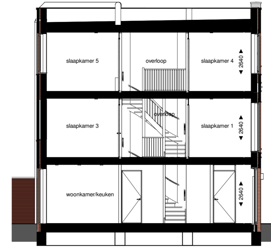
doorsnede 1 : 100
