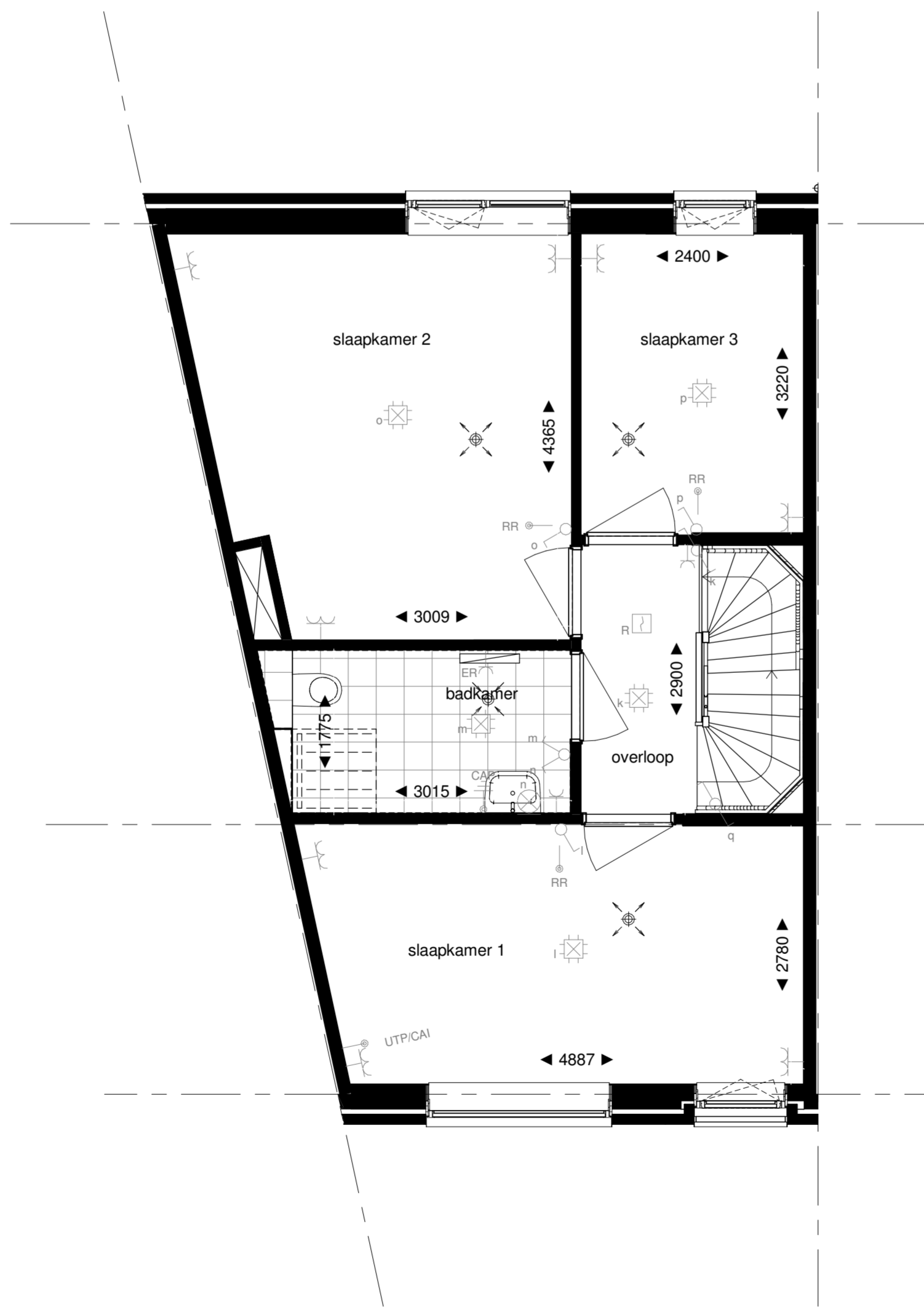
1e verdieping 1 : 50
