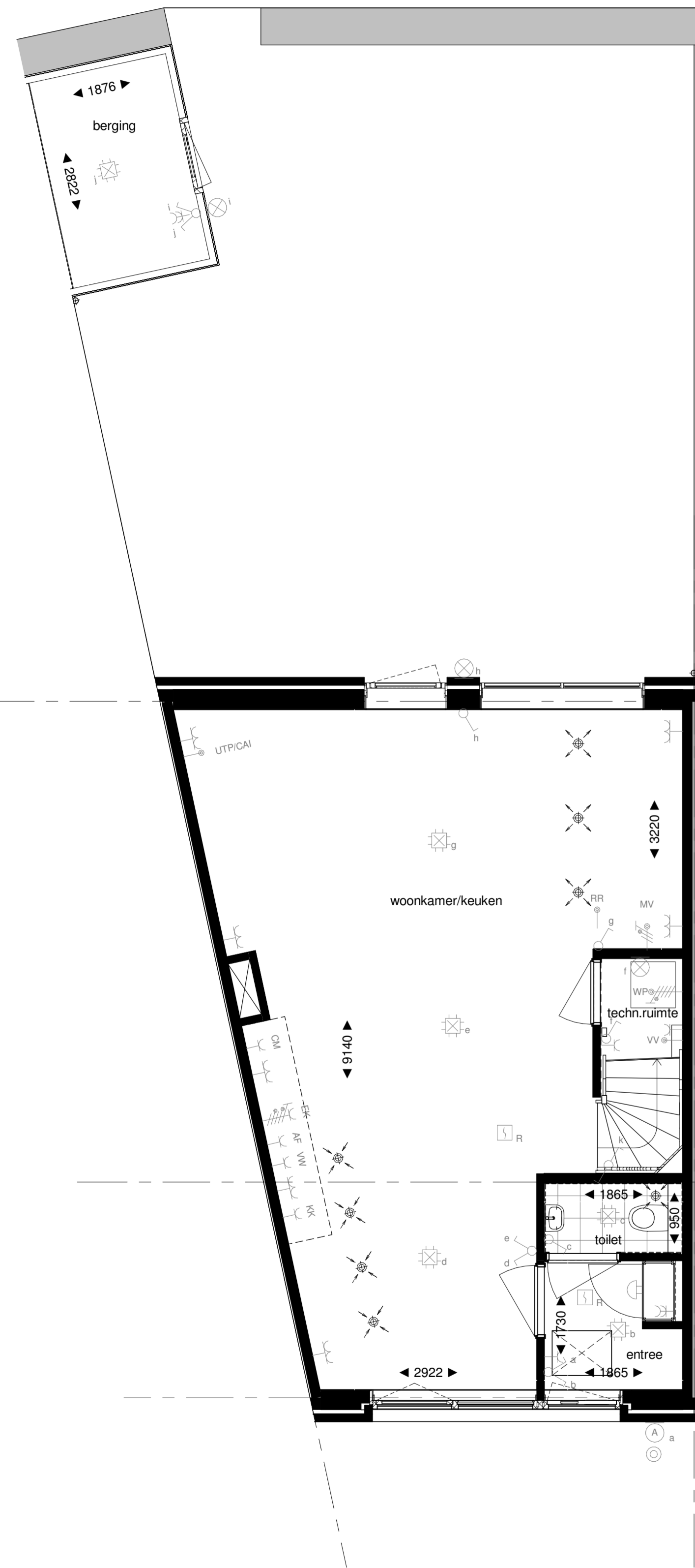
begane grond 1 : 50
